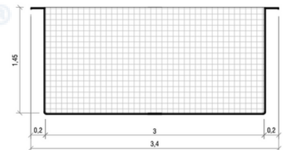
CORTE TRANSVERSAL BB. ESCALA 1:50
