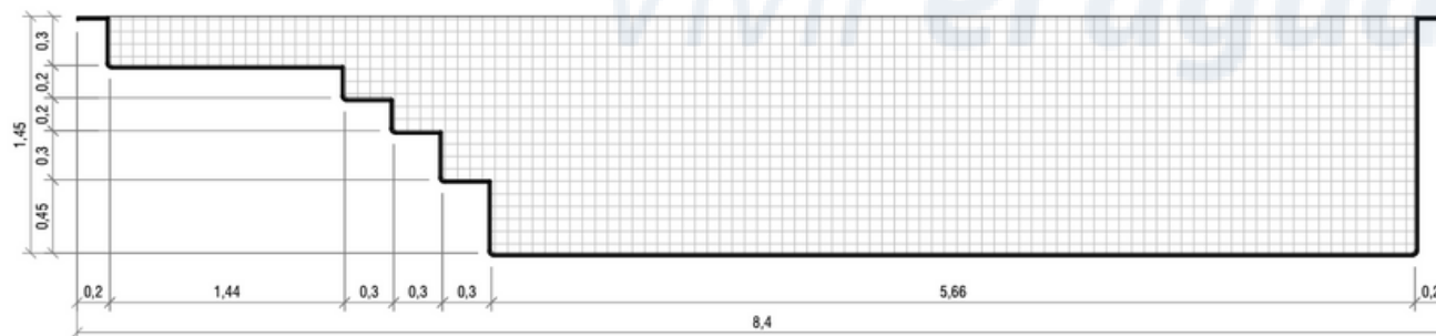
CORTE LONGITUDINAL AA. ESCALA 1:50
