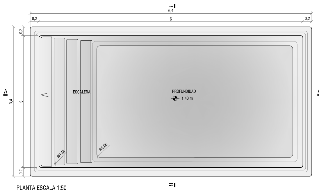
PLANTA ESCALA 1:50
