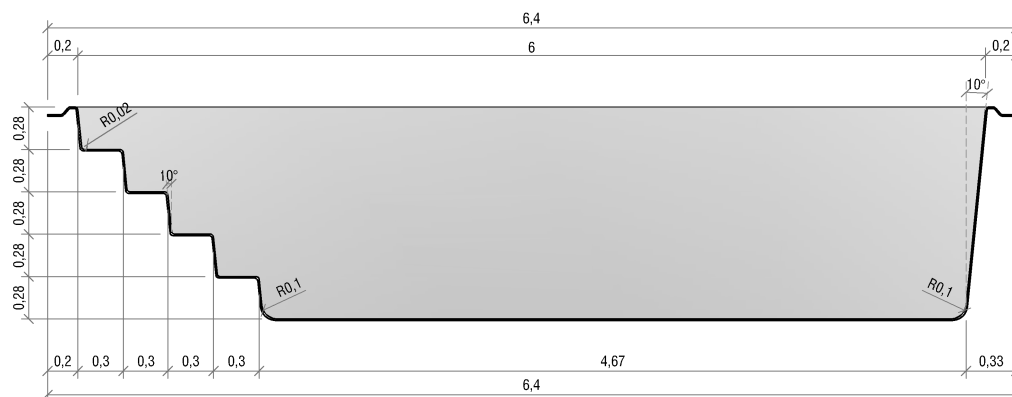
CORTE LONGITUDINAL AA. ESCALA 1:50
