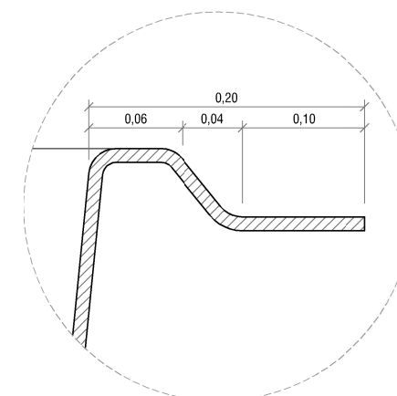
DETALLE D1. ESCALA 1:50
